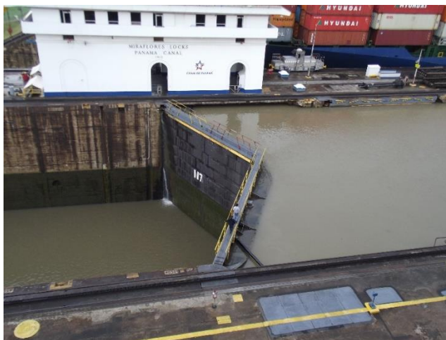
Eclusa Miraflores. Canal do Panamá, Panamá. Foto de Samuel Sembalista Haurelhuk, 2013.
