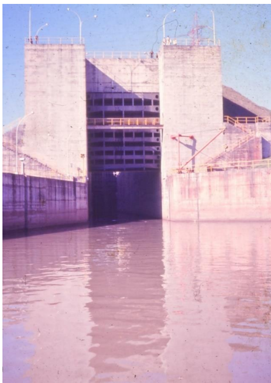
Guia de acesso a eclusa de Promissão. São Paulo, Brasil. Foto de Carlos Eduardo D'Almeida, 1979.
