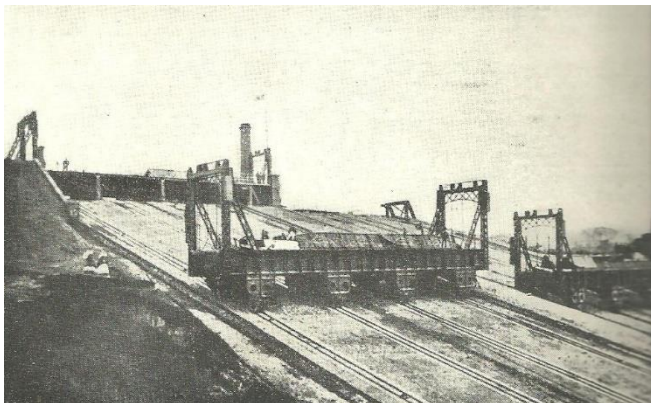
Foto 1/2. Duas das poucas fotos do plano inclinado transversal de Foxton.
