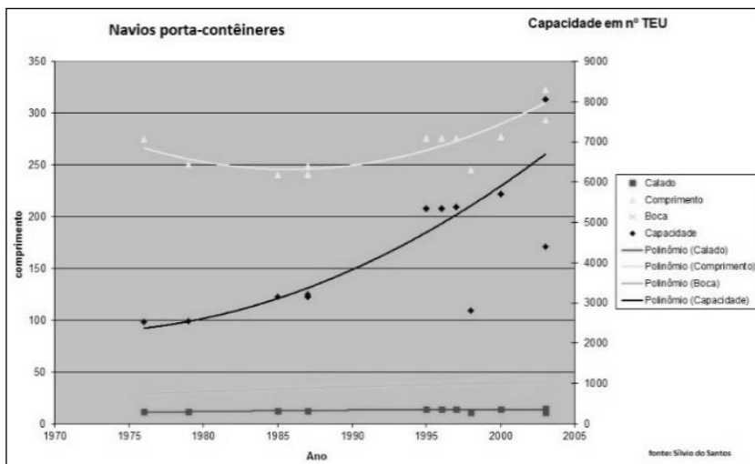
Evolução do porte dos navios porta-contêineres. Elaboração: Sílvio dos Santos, 2012.
