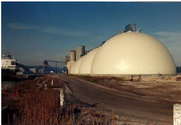
Silos para grãos. Porto de Rouen, França. Foto de Sílvia dos Santos, 1991.
