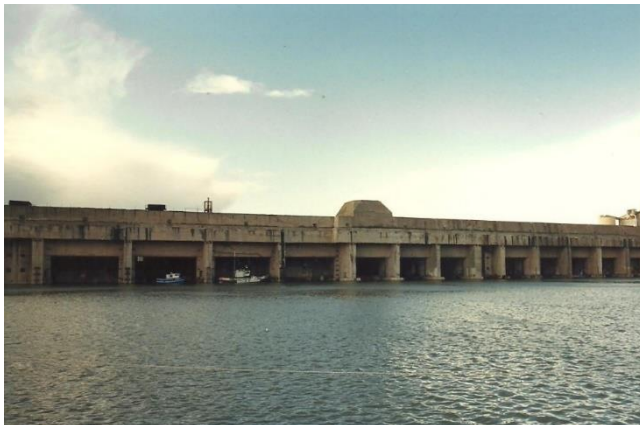
Garagem marítima dos submarinos alemães u-boots. Porto de Lorient, França. Foto de Sílvio dos Santos, 1991.
