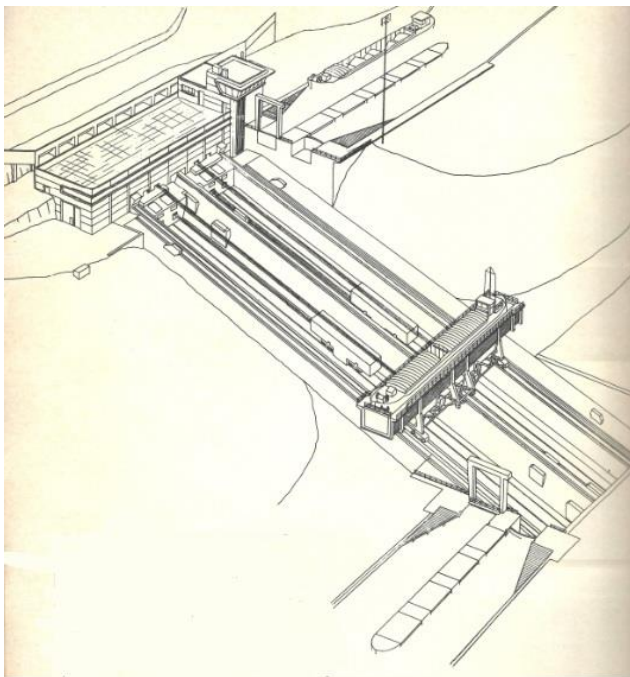
Perspectiva do plano inclinado transversal de Arzwiller, Saint Louis. Fonte: Service de la Navigation de Strasbourg. Revue Navigation, Ports et Industries – 25/06/1970.
