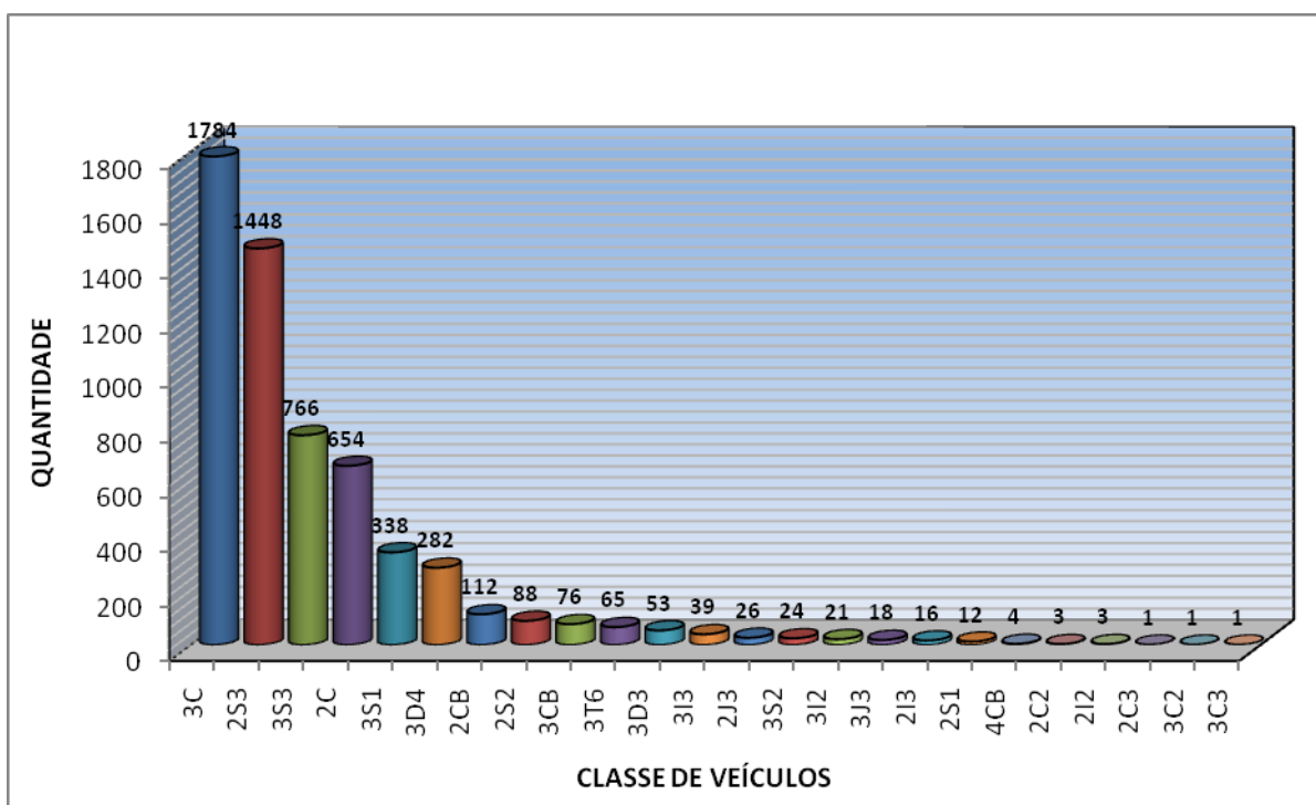
Figura 4 – Total de Veículos por Classe, segundo classificação do DNIT.
