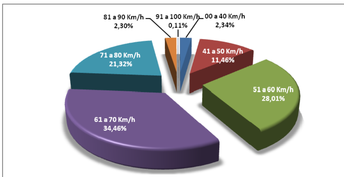
Figura 5 –Velocidade dos veículos de carga representativos da frota (3C, 2S3, 3S3 e 2C)
